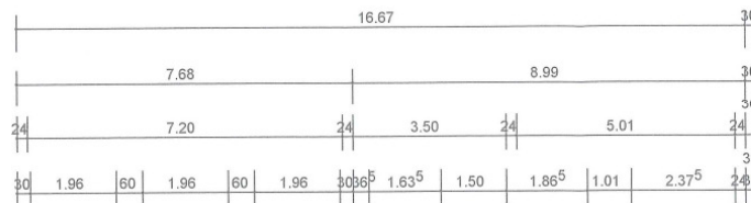
Schnitt A-A
